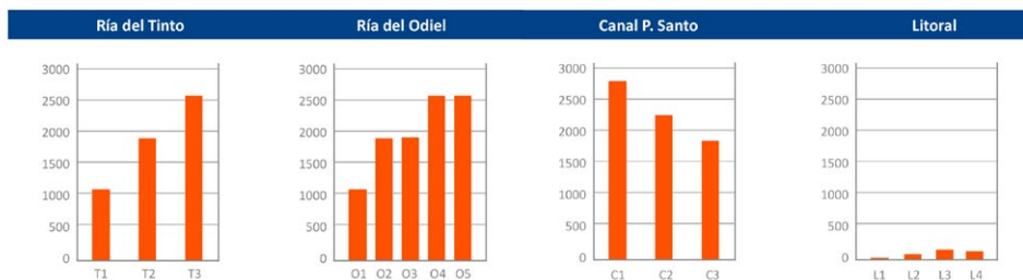
Figura 4. Evolución de las concentraciones de cobre en los sedimentos y aguas de la Ría de Huelva. Fuente: Memoria AIQBE 2021
